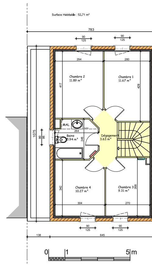
PLAN ETAGE
