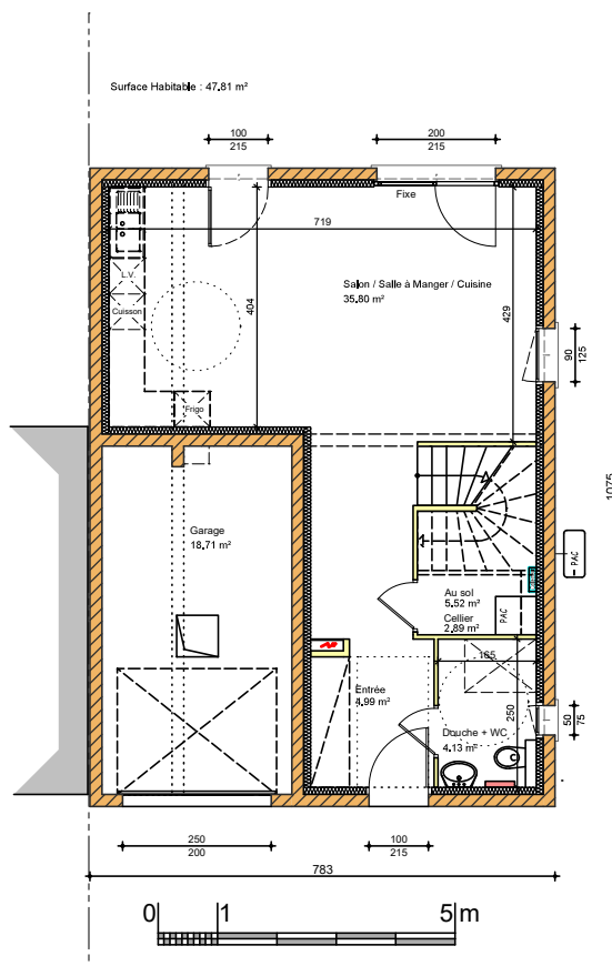
PLAN REZ DE CHAUSSEE
