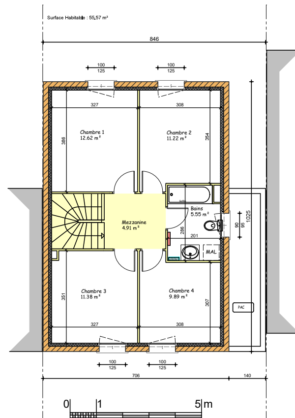
PLAN ETAGE
