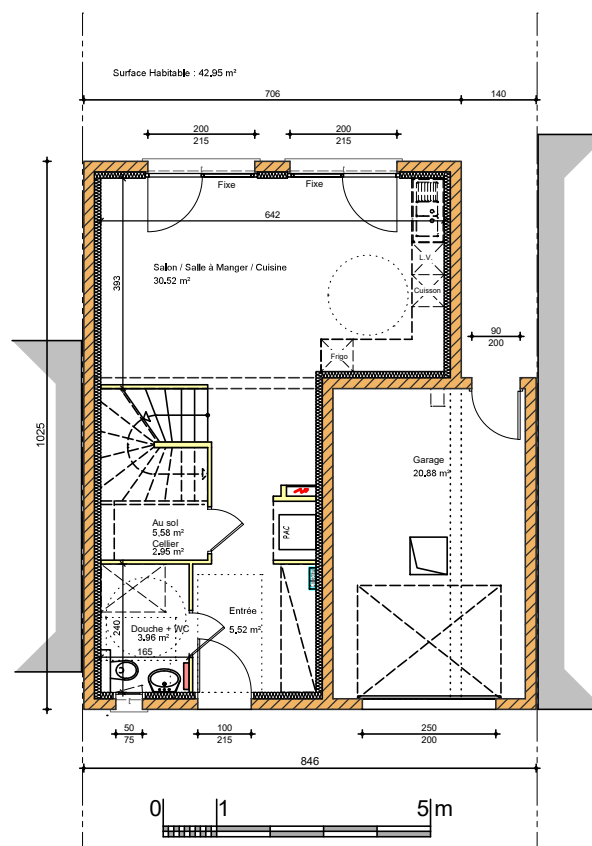
PLAN REZ DE CHAUSSEE
