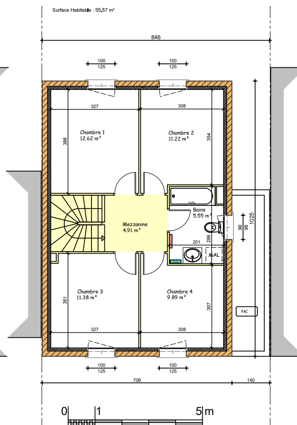
PLAN ETAGE
