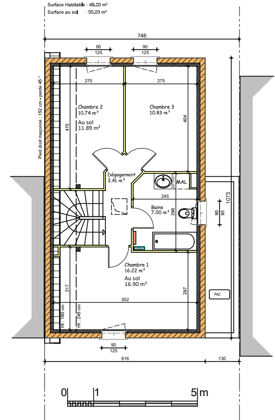
PLAN ETAGE
