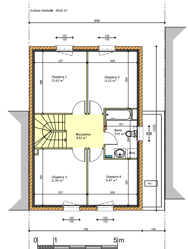
PLAN ETAGE
