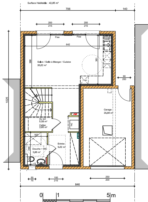
PLAN REZ DE CHAUSSEE
