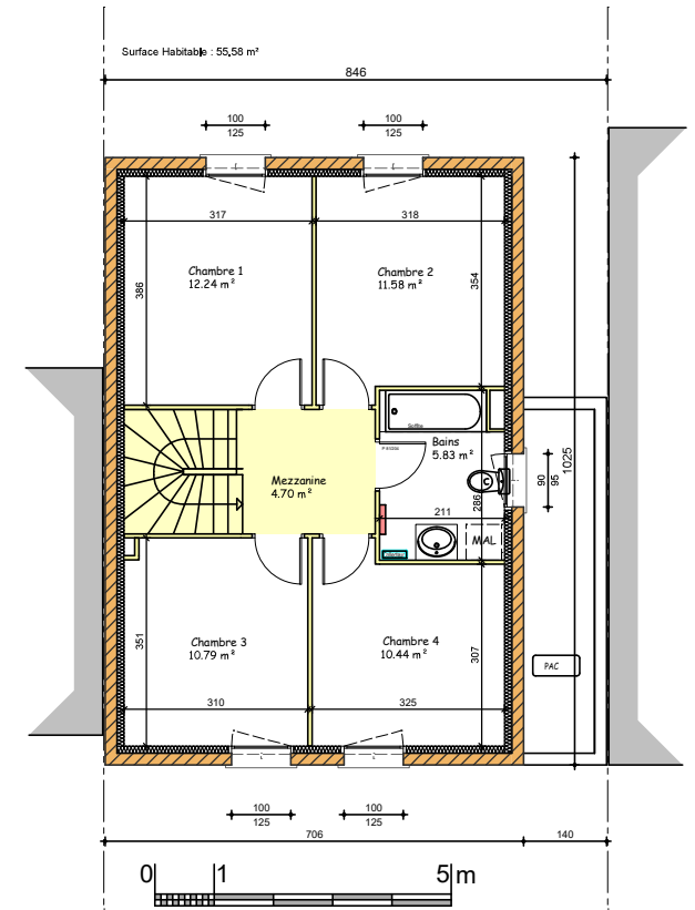
PLAN ETAGE
