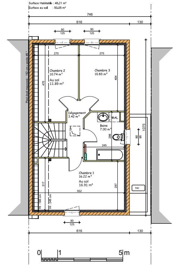
PLAN ETAGE
