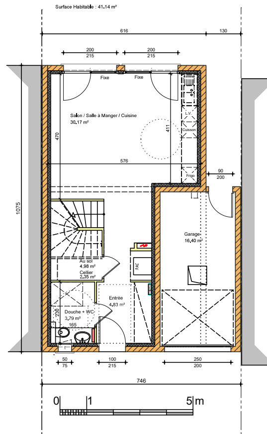
PLAN REZ DE CHAUSSEE
