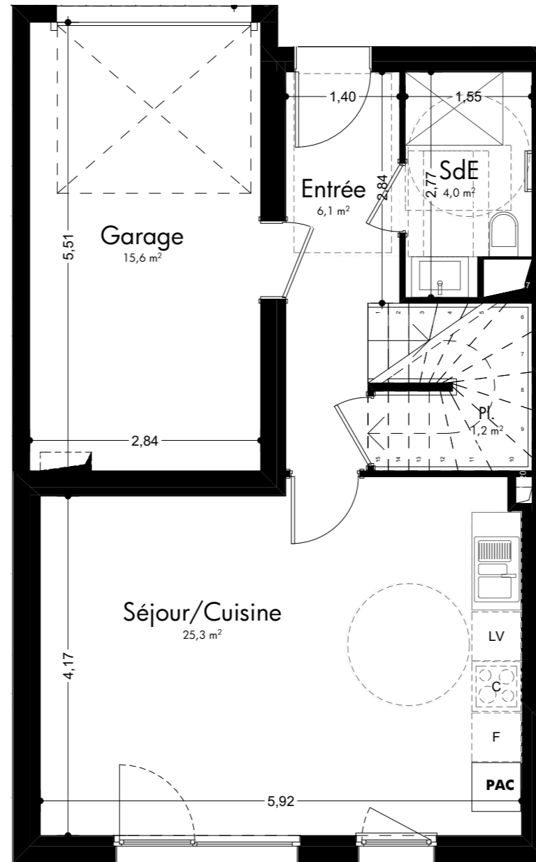
PLAN REZ-DE-CHAUSSEE
