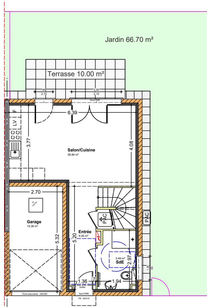
PLAN DU REZ DE CHAUSSEE AVEC JARDIN
