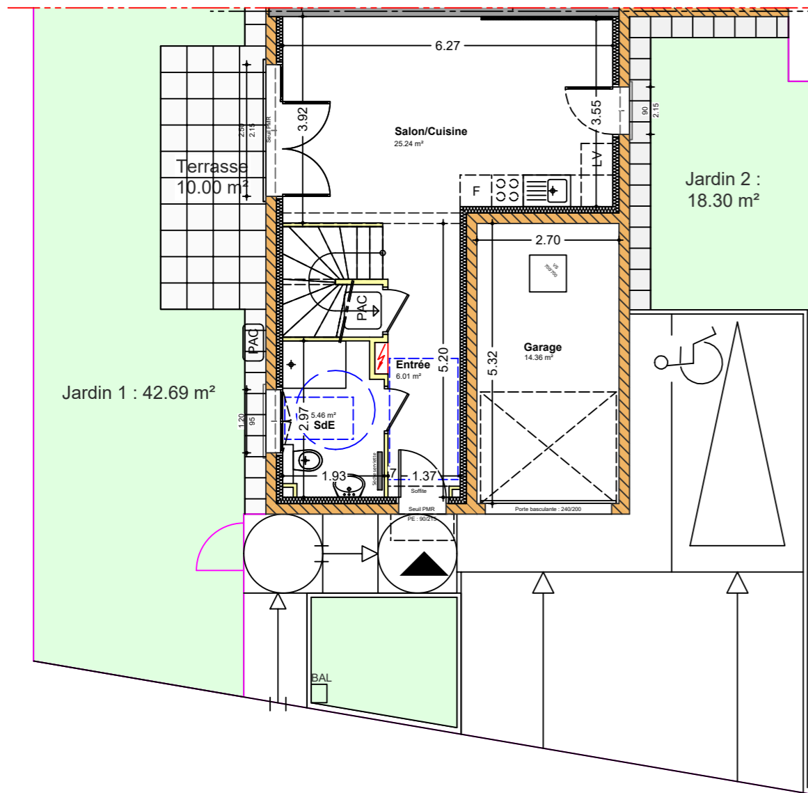
PLAN DU REZ DE CHAUSSEE AVEC JARDIN
