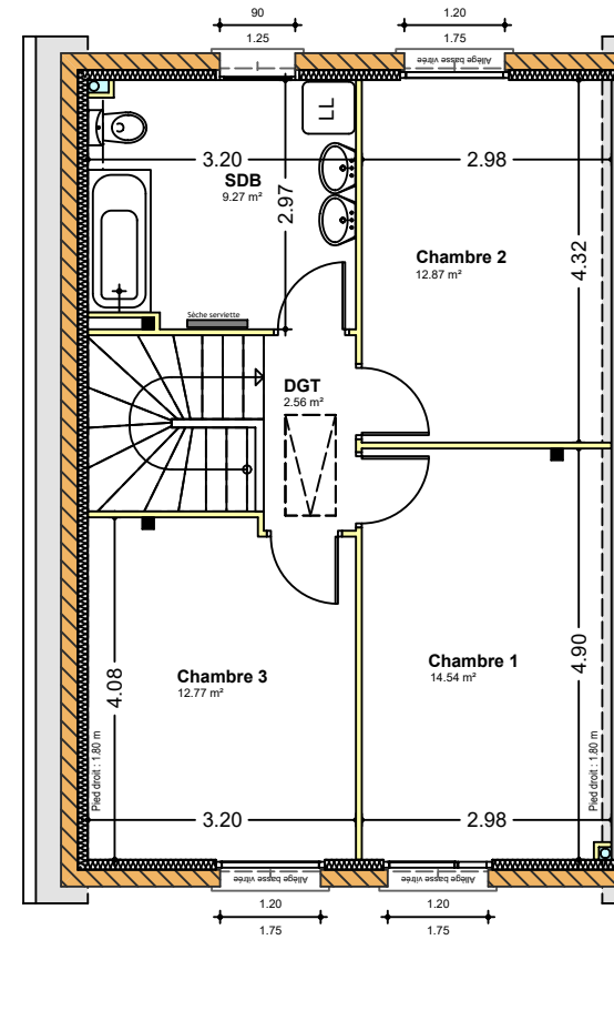
PLAN DE L'ETAGE
