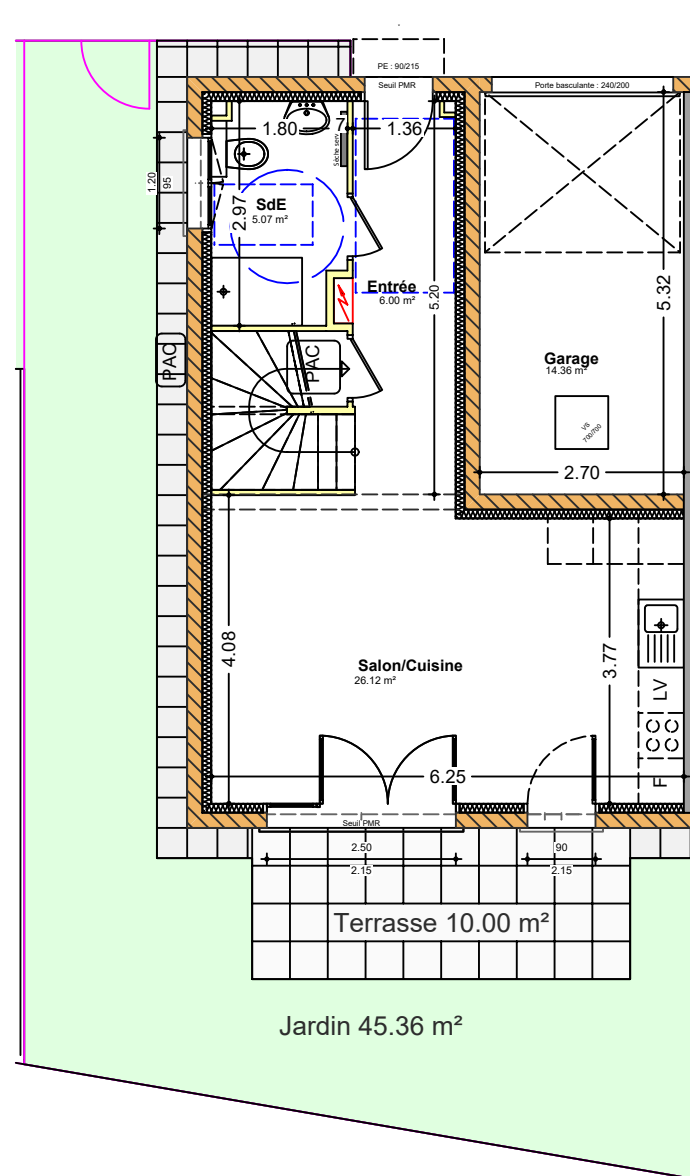
PLAN DU REZ DE CHAUSSEE AVEC JARDIN
