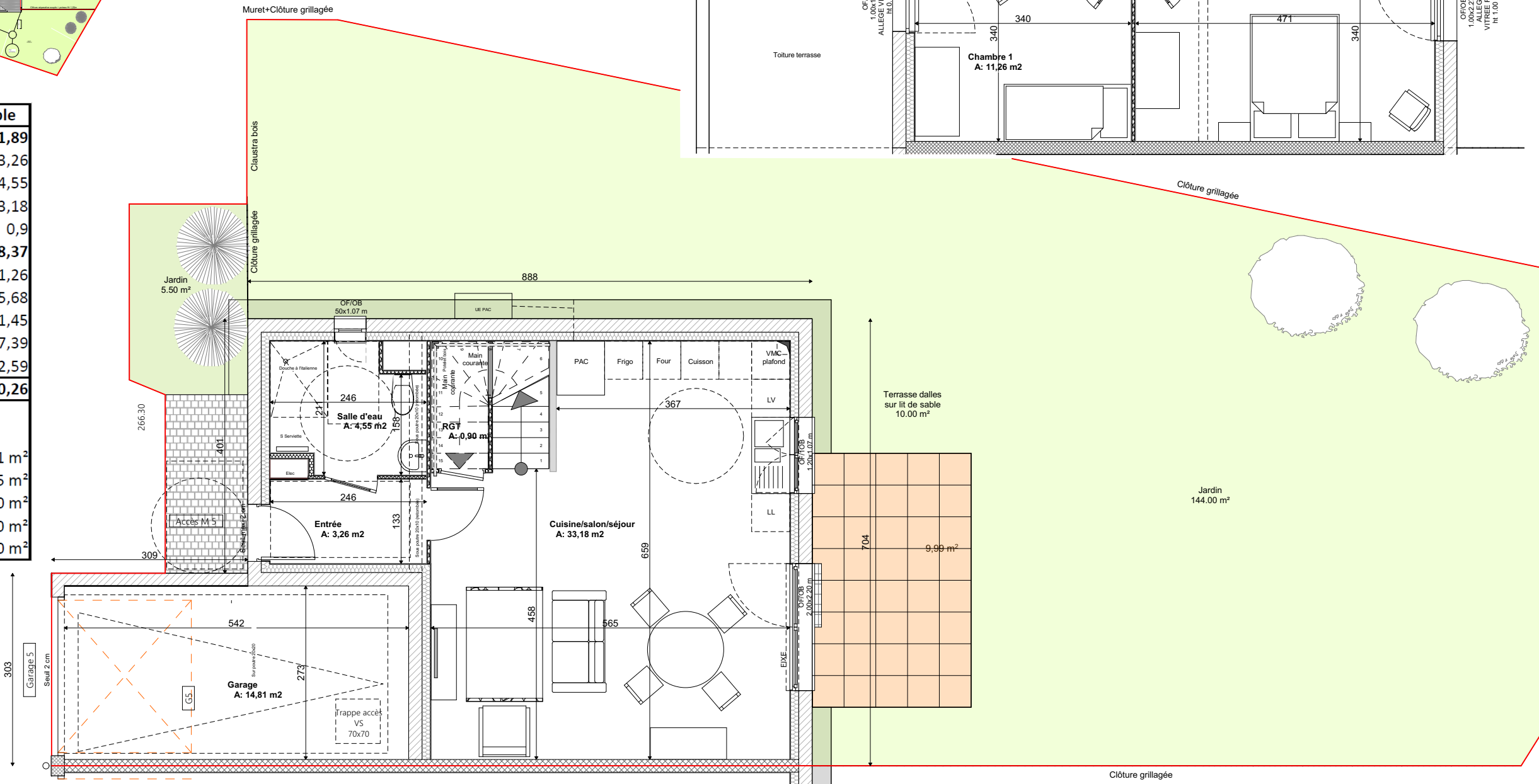
Plan du Rez-de-chaussée
