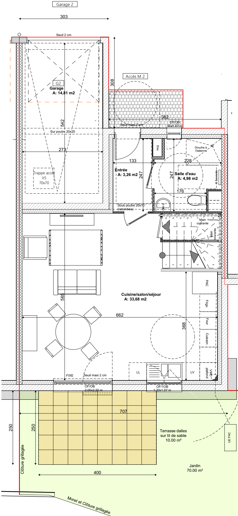
Plan du Rez-de-chaussée
