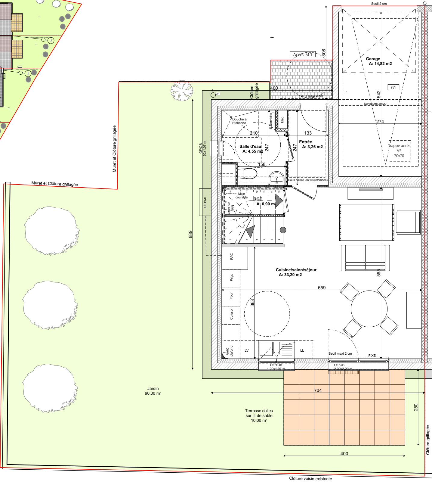
Plan du Rez-de-chaussée
