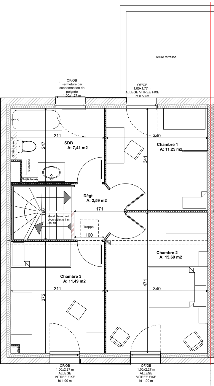
Plan de l'étage
